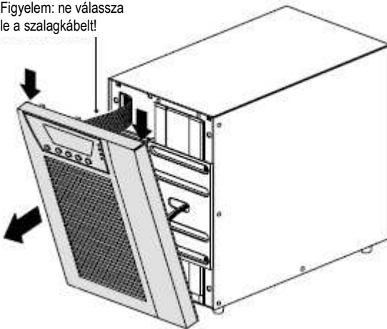
25. ábra: Az UPS előlapjának eltávolítása
