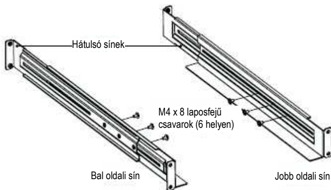
4. ábra: A sín összeszerel ése
