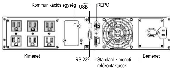
18. ábra: Kommunikációs lehetőségek és vezérlőterminálok (PW9130L1000R-XL2U modell)
